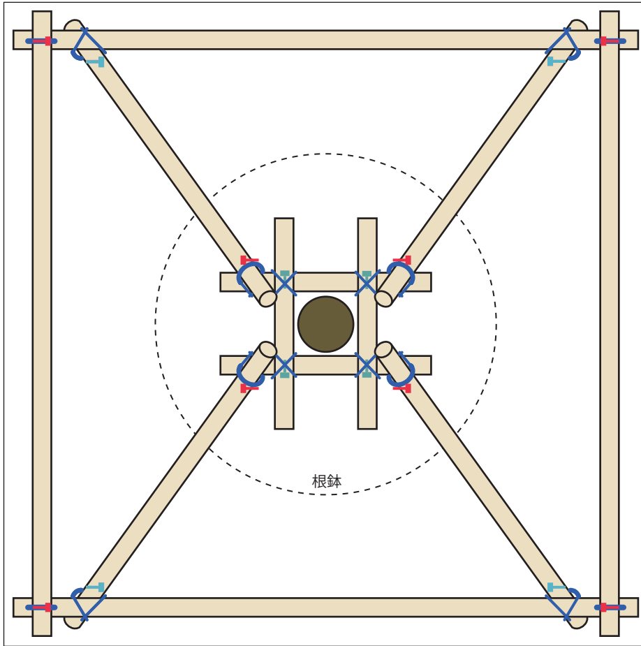
ラッピングサポート平面図
